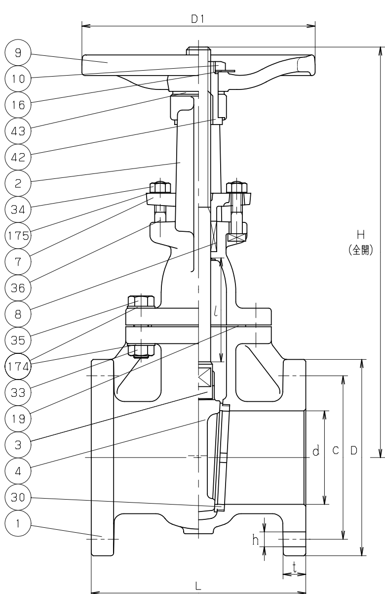
寸法表
